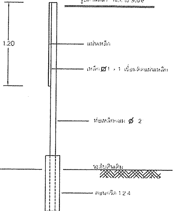
รูปด้านเหล็ก NOT to Scale
