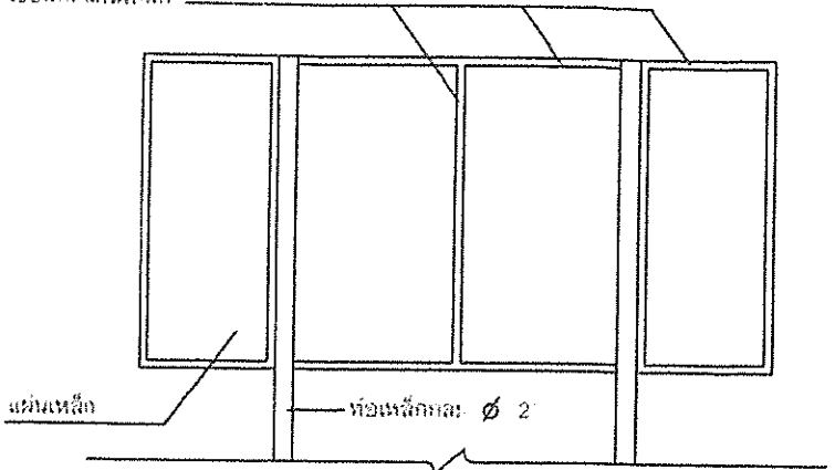
รูปด้านเหล็ก NOT to Scale
